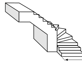
④ Escalier à 90° sans palier
